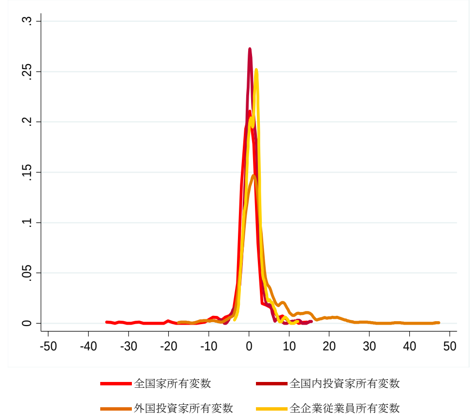
(b) t 値
